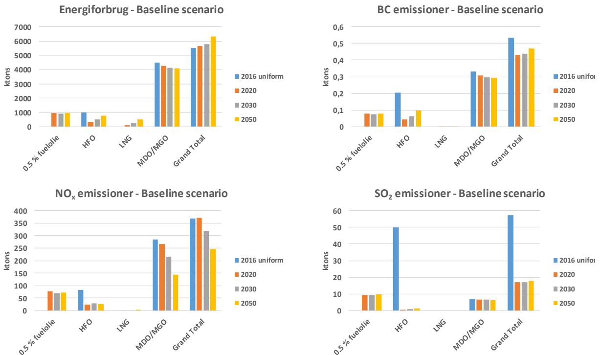
Figur DS 3 Totaler for energiforbrug (massebasis), NO x , SO 2 og BC emissioner beregnet for 2016 (ensartet gitterfordelt) og for 2020, 2030 og 2050 i Baseline scenariet.
