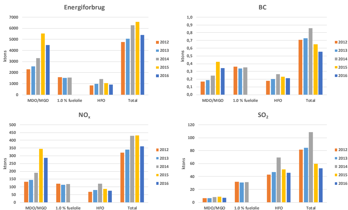
Figur DS 1 Totaler for energiforbrug (massebasis), NO x , SO 2 og BC emissioner beregnet i 2012-2016.
