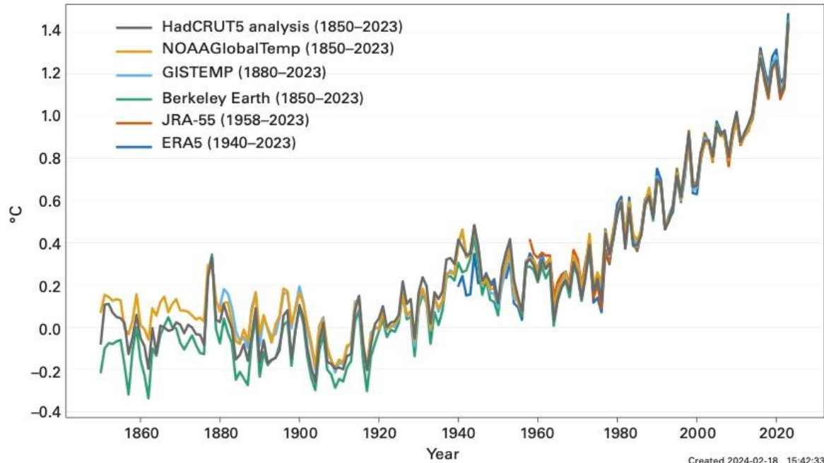
WMO, 2024
