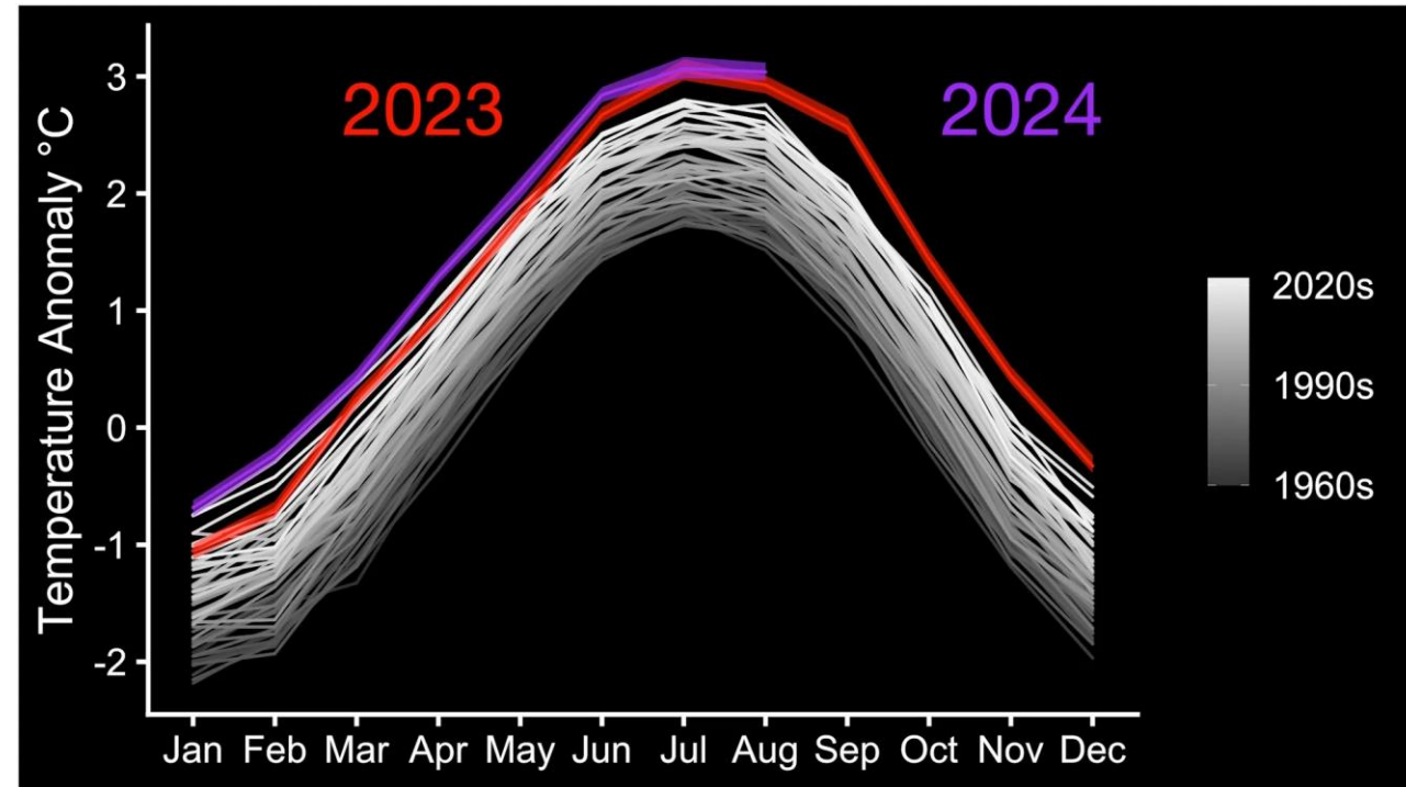
NASA GISS, 2024
